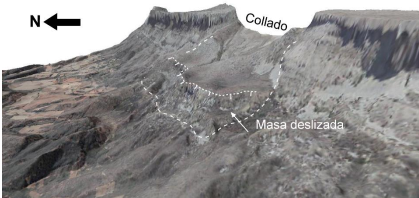
Figura 6: Deslizamiento de la Peña Villanueva. Nótese que los acantilados de la parte superior han bajado de cota en la masa deslizada.
