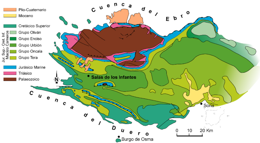
Figura 3: Esquema geológico del Macizo de Cameros y Demanda.
